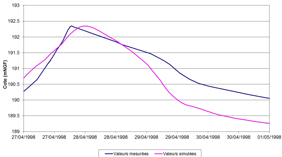
Station hydrométrique de Dissangis - Crue Avril 1998
