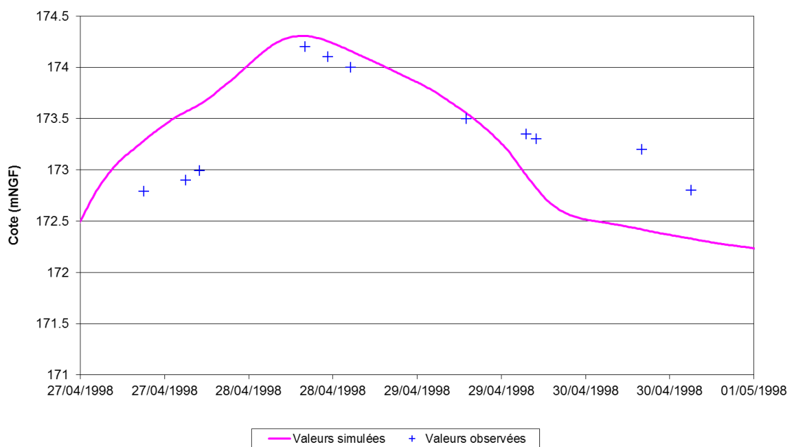
Echelle de Noyers - Crue Avril 1998
